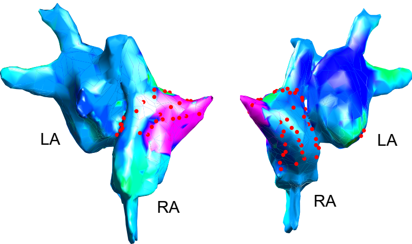
Tikh
