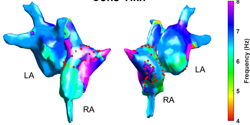
Cons-Tikh
